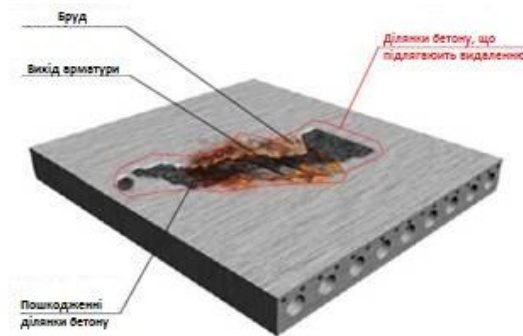
Рис. 1. Корозія бетону
