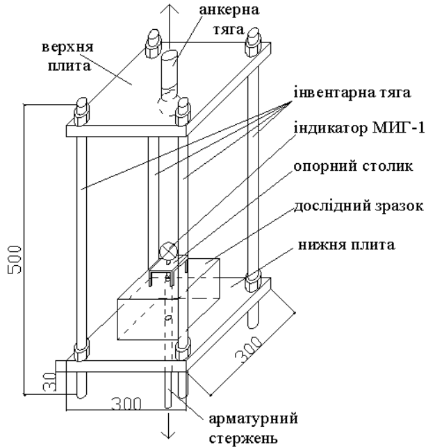
Рис. 1. Схема висмикування арматури з призм в устаткуванні розривної машини
