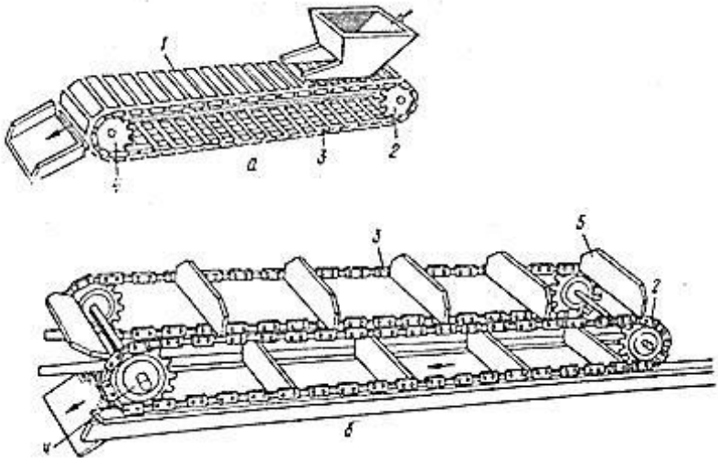
Рис. 1. – Конвеєри з ланцюговим тяговим органом [3] : 1 – пластина; 2, 4 – натяжна і привідна зірочки; 3 – ланцюг; 5 – скребок
