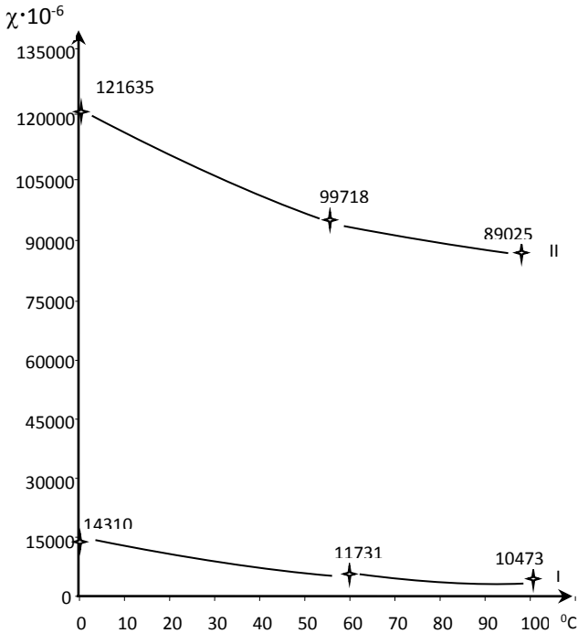
Рис. 2. Залежності \chi_m від температури парамагнітних сполук:
