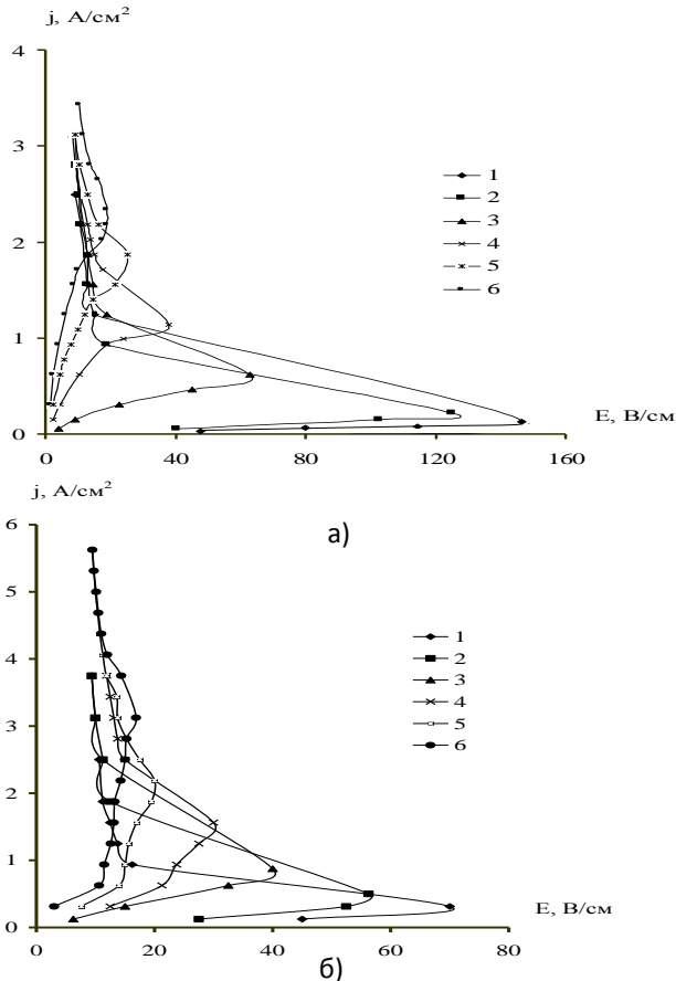
Рис. 3. Залежності j=f(E) при 77 К для зразків CdSb(Te), вирізаних паралельно (а) та перпендикулярно (б) до осі росту кристала, при різній інтенсивності освітлення I , відн.од.: 1 – 0; 2 – 0,25; 3 – 0, 5; 4 – 1; 5 – 2; 6 – 4
