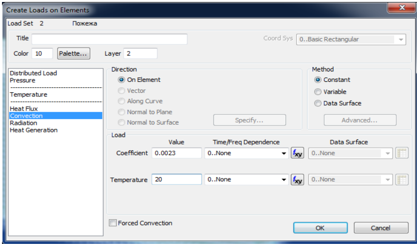
Рис.7. Діалогова панель «Create Loads on Elements» для задання навантаження на весь елемент (тут - тепловіддачі)
