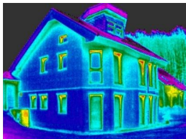
Рис.2 Тепловтррати "пасивного будинку
