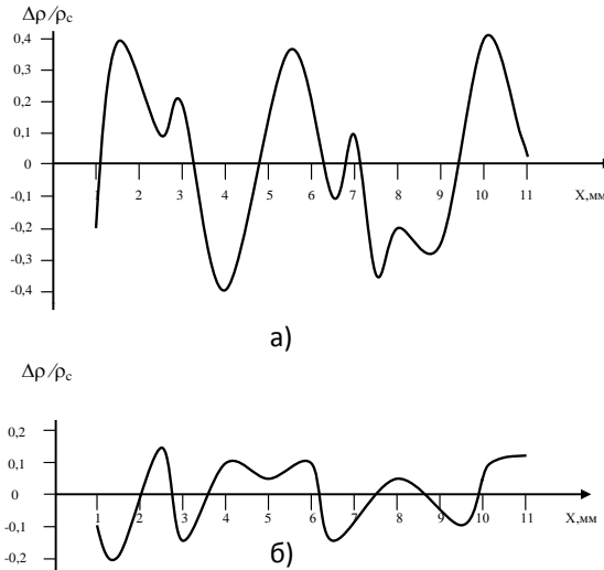
Рис. 1. Відносні відхилення питомого опору від середнього значення для зразків CdSb(In), вирізаних: а) паралельно; б) перпендикулярно до осі росту кристала
