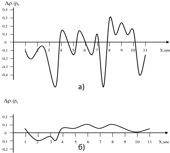
Рис. 1. Відносні відхилення питомого опору від середнього значення для зразків CdSb(In), вирізаних: а) паралельно; б) перпендикулярно до осі росту кристала
