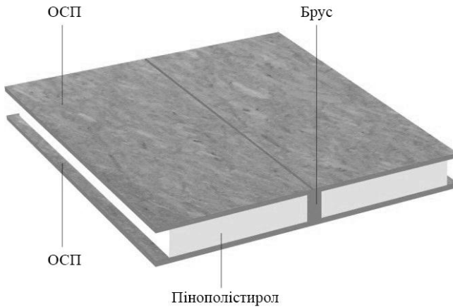
Рисунок 1. Конструкція структурно-ізольованої панелі.
