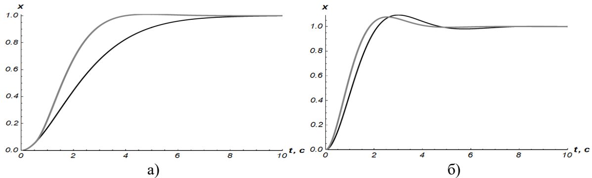
Рисунок 1. Графіки, які відповідають відпрацюванню уставки для об'єкта регулювання із передаточною функцією G_1(s) та методів налаштування ПІ-регулятора: а) AMIGO; б) Скогестада
