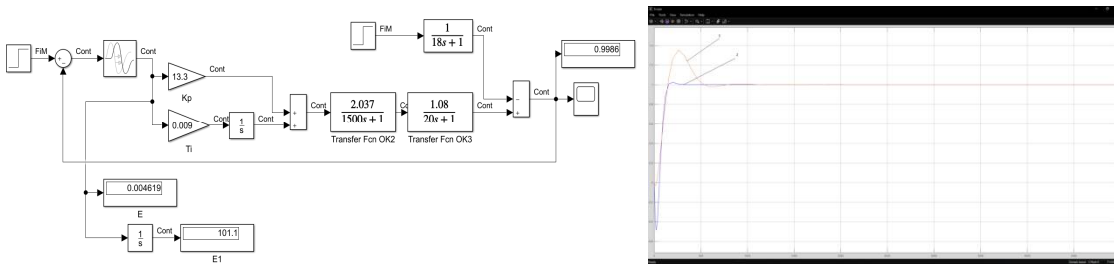
Рисунок 3. Структурна схема моделювання САР з ПІ-регулятором та її графік перехідного процесу:
