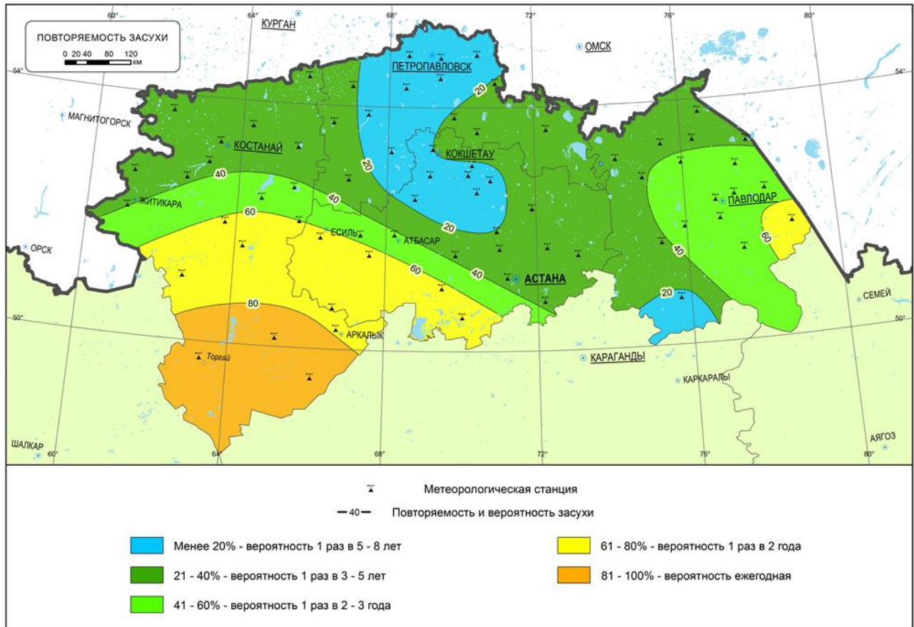
Рис. 2 – Повторяемость атмосферной засухи в Северном Казахстане
