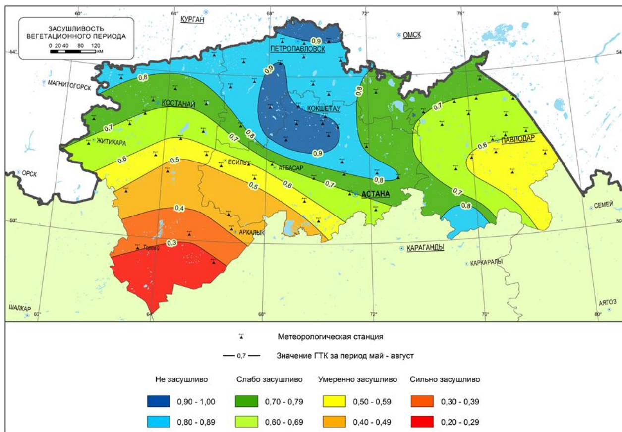
Рис. 1 – Засушливость вегетационного периода в Северном Казахстане
