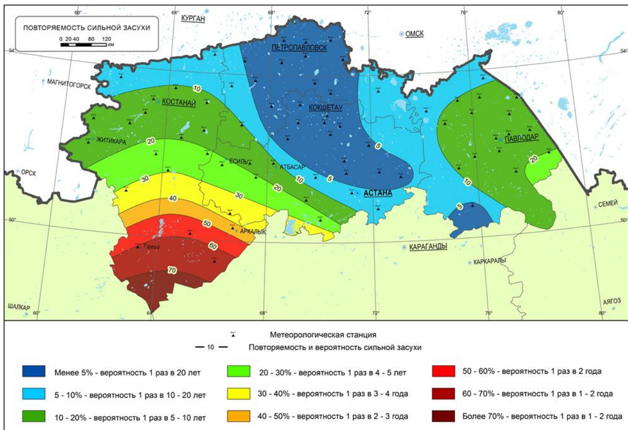
Рис. 3 – Повторяемость сильной засухи в Северном Казахстане
