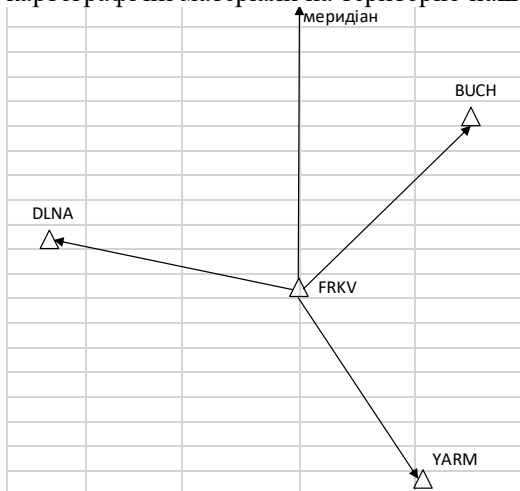
Рис.1 - Схема розміщення постійних станцій
