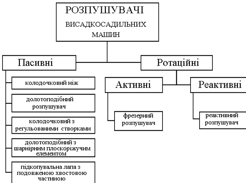
Рисунок 1 – Класифікація розпушувачів
