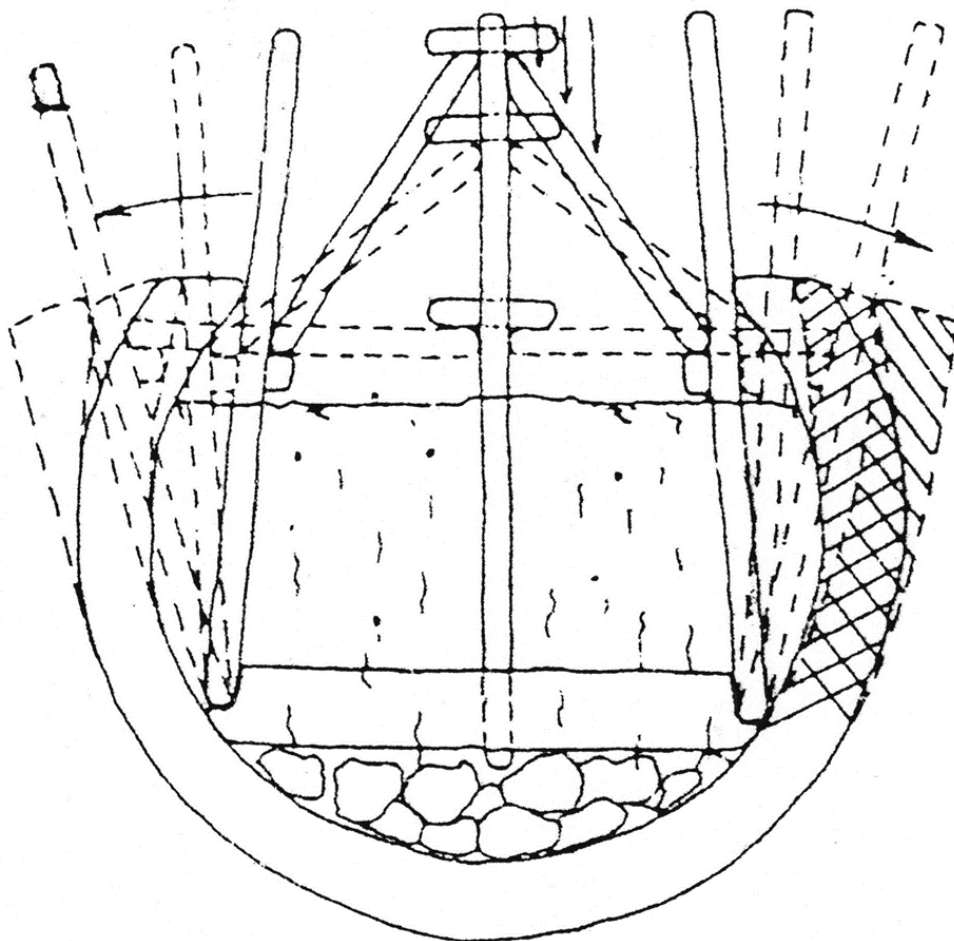
Рис. 11. Поперечний розріз човна-довбанки, технологічний процес розводу бортів
